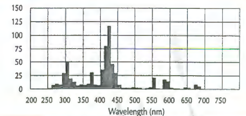
Spectrum: Ga 3 / Ga 3 InI, Hg
