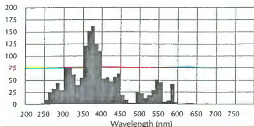
Spectrum: Fe 2 Co 2 TlI, Hg
