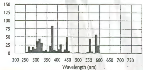
Spectrum: Hg
